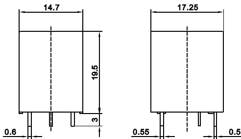
外形尺寸
