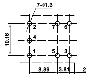
安装孔位图 (底视图)
